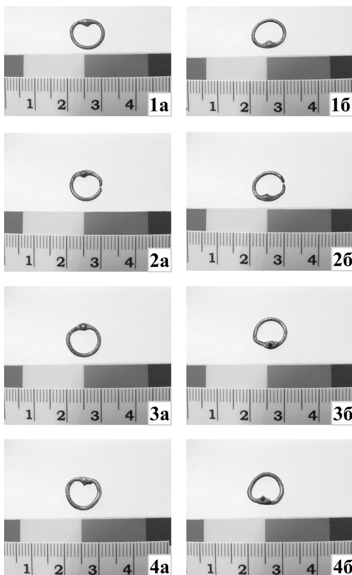
Образцы клепаных колец кольчуги ЧОКМ ОФ-448/2: 1–2 — с прямоугольной заклепкой; 3–4 — с круглой заклепкой.
