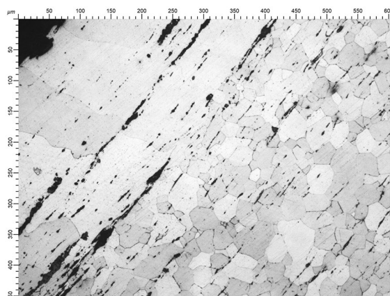
Кольцо № 2: 1 — общий вид шлифа, \times 50 ; 2 — заклепка, \times 100 ; 3 — микроструктура, \times 200 (феррит и шлаковые включения); 4 — микроструктура, \times 200 (граница участков мелкозернистого и крупнозернистого феррита и шлаковые включения). Фото А. Ю. Щедриной
