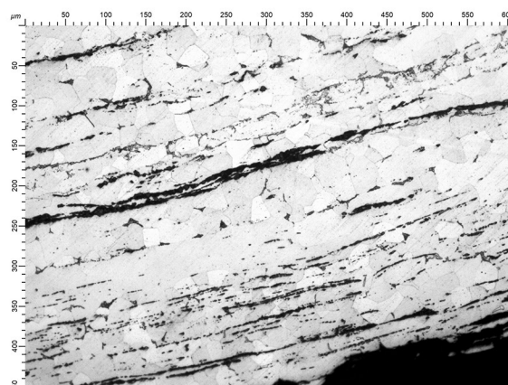
Кольцо № 1: 1 — общий вид шлифа, \times 50 ; 2 — заклепка, \times 100 ; 3 — микроструктура, \times 200 (феррит и крупные шлаковые включения); 4 — микроструктура, \times 200 (феррит, незначительные включения перлита и шлаковые включения). Фото А. Ю. Щедриной
