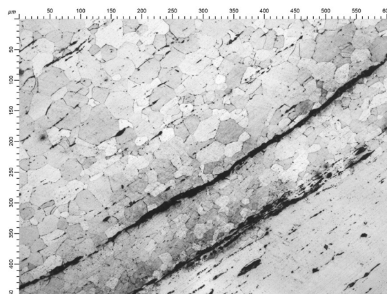
Кольцо № 2: 1 — общий вид шлифа, \times 50 ; 2 — заклепка, \times 100 ; 3 — микроструктура, \times 200 (феррит и шлаковые включения); 4 — микроструктура, \times 200 (граница участков мелкозернистого и крупнозернистого феррита и шлаковые включения). Фото А. Ю. Щедриной
