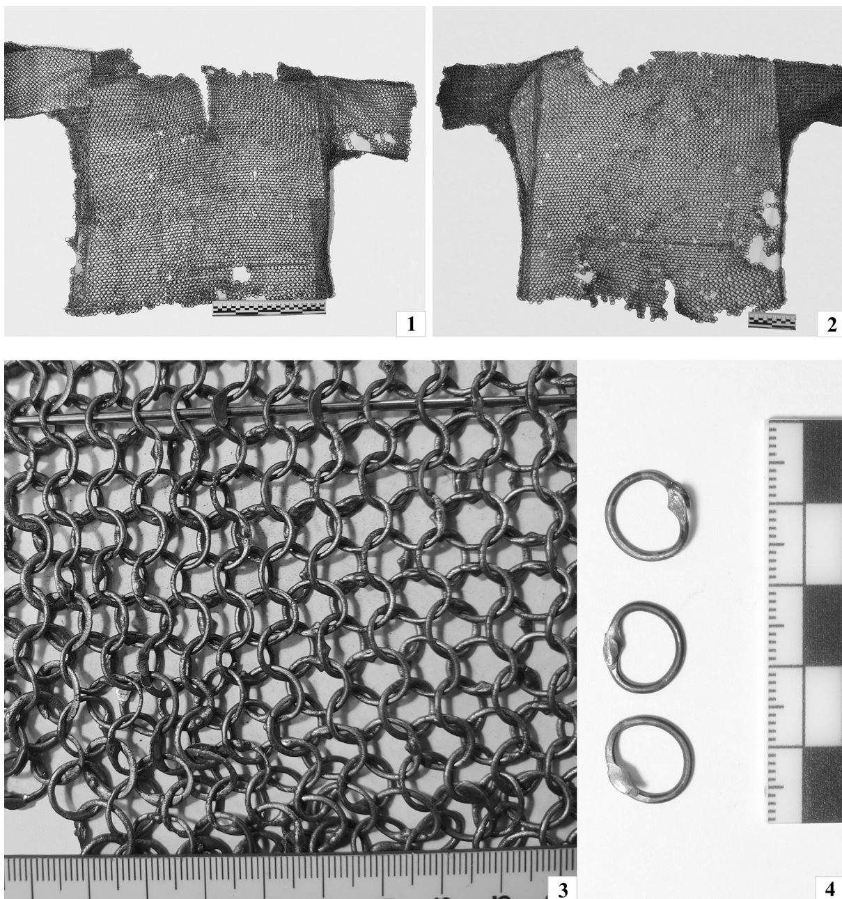
Кольчуга ЧОКМ ОФ-448/2 после расчистки, консервации и локального монтажа новодельных колец: 1 — общий вид лицевой стороны; 2 — общий вид оборотной стороны; 3 — фрагмент полотна; 4 — образцы новодельных колец. Фото А. Д. Шапиро
