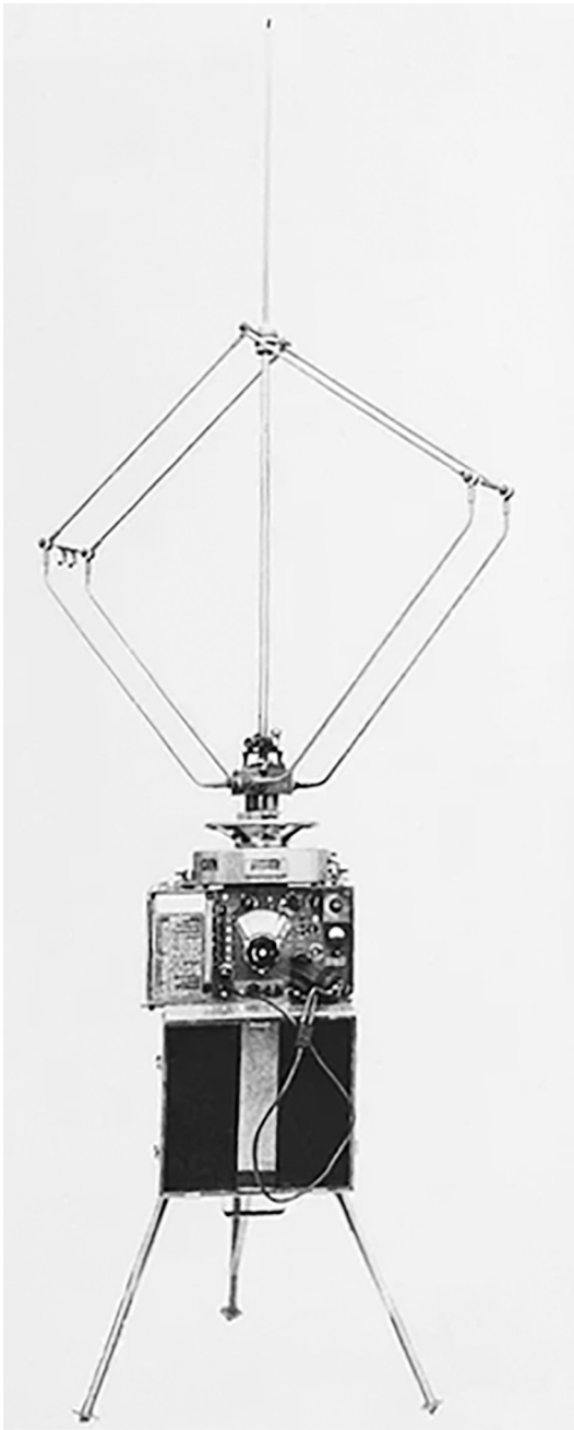
Радиопеленгатор со штыревой антенной производства Каслинского радиозавода № 193
