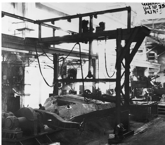
Сварка корпуса танка Т-10 на заводе № 78 (Станкомаш)
