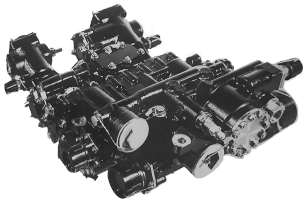
Регулятор подачи топлива для ракет РПТ-1А производства Симского механического завода № 132 (регулирует расход топлива двигателя ракеты в зависимости от заданной траектории; производит корректировку подачи топлива по высоте полета, температуре воздуха и другим внешним факторам, влияющим на режим работы двигателя)
