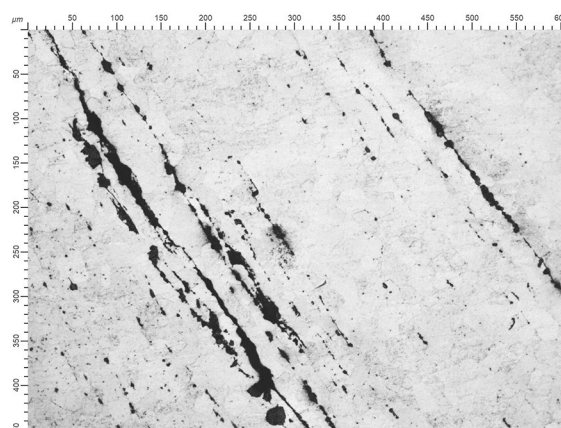
Кольцо № 3: 1 — общий вид шлифа, \times 50 ; 2 — заклепка, \times 100 ; 3 — микроструктура, \times 200 (феррит и шлаковые включения); 4 — микроструктура, \times 200 (феррит, шлаковые включения, край заклепки). Фото А. Ю. Щедриной
