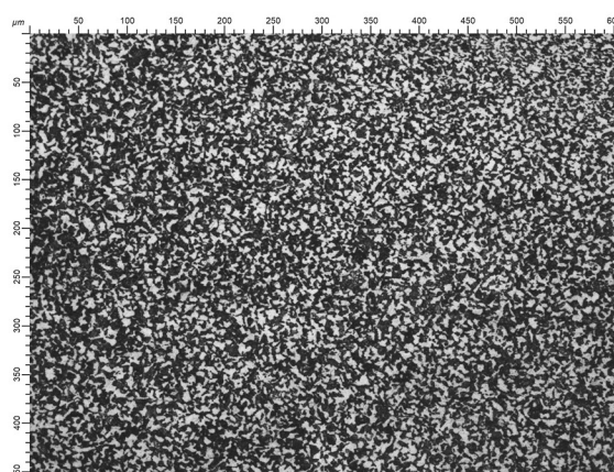
Кольцо № 4: 1 — общий вид шлифа, \times 50 ; 2 — заклепка, \times 100 ; 3 — микроструктура, \times 200 (феррит и перлит — средне науглероженный участок); 4 — микроструктура, \times 200 (феррит и перлит — сильно науглероженный участок). Фото А. Ю. Щедриной
